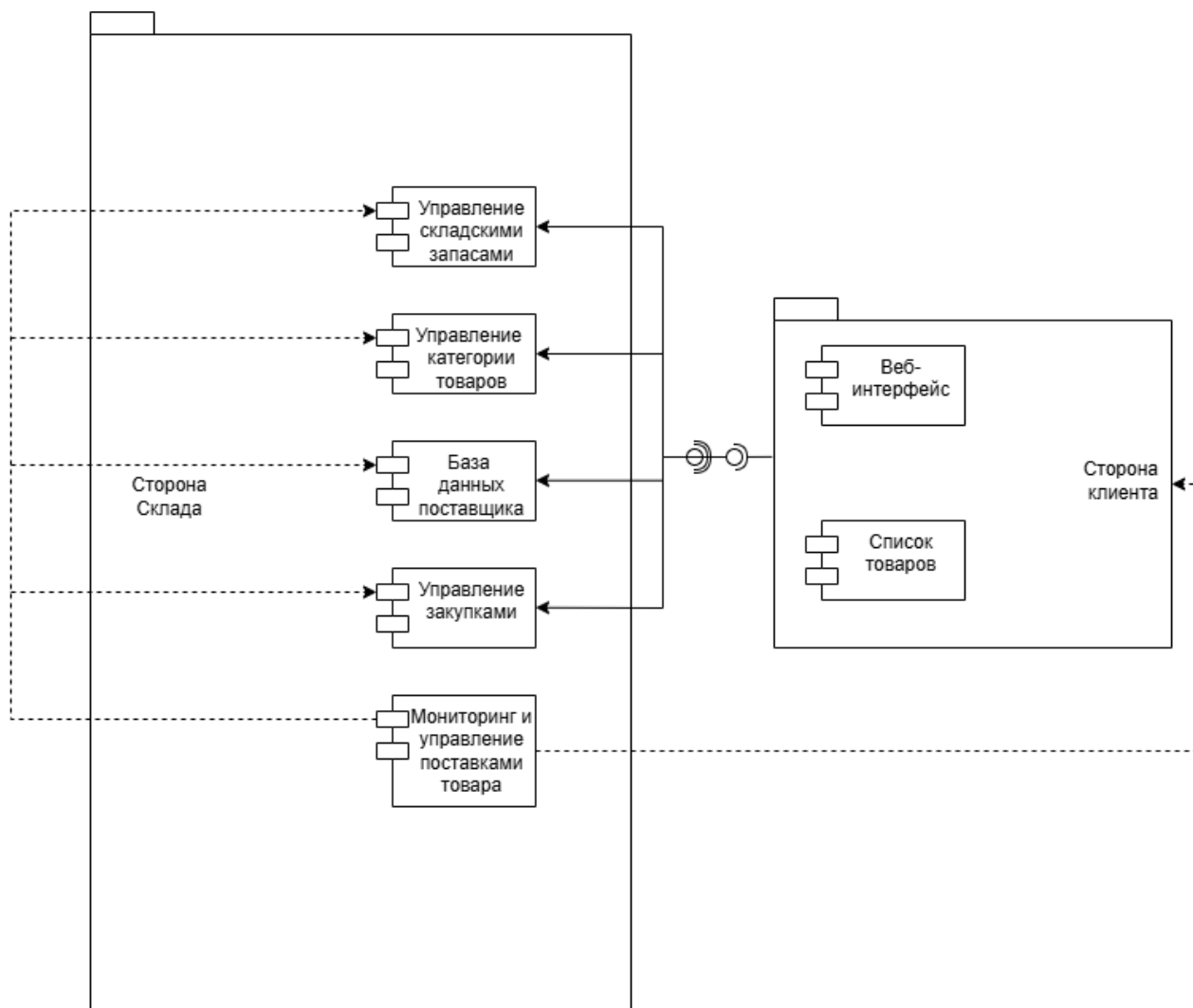
Рисунок 1 – Диаграмма компонентов
