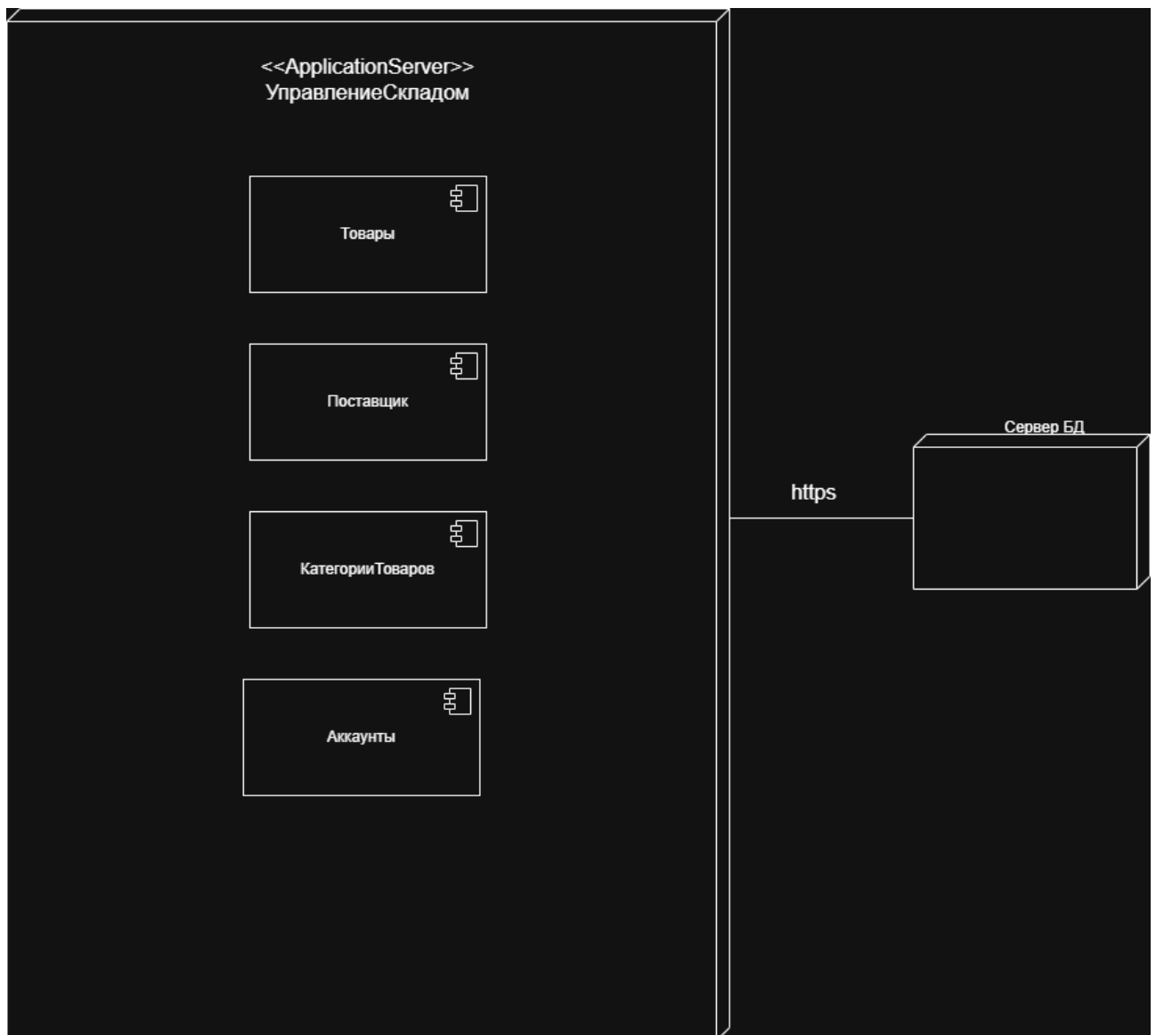
Рисунок 2 – Диаграмма развертывания
